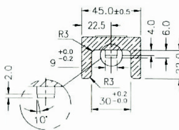
VISTA LATERAL CORTE B-B
